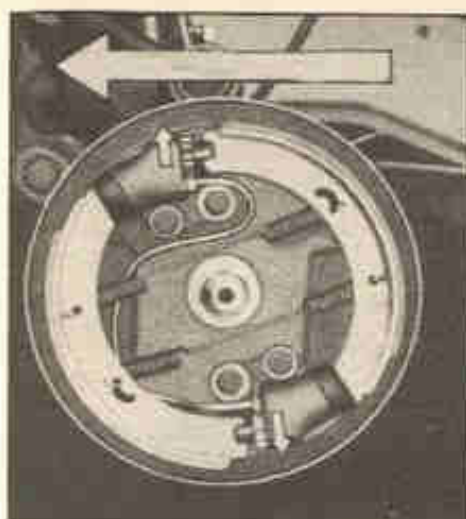
Fig. 10-R — Prato de freio das rodas dianteiras dos utilitários. Cada sapata é acionada por um cilindro. A seta horizontal mostra a frente do veículo. As setas menores mostram os sentidos em que os reguladores devem ser girados para aproximar as sapatas do tambor de freio. Nos modelos alemães antigos, há um só cilindro de roda e os reguladores se encontram na parte inferior, ligeiramente afastados para a parte de trás.
