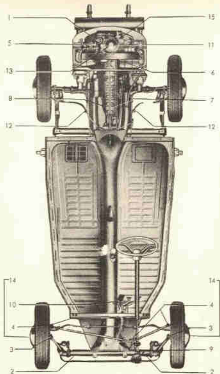
Plano de lubrificação para o sedan e o Karmann Ghia. A ilustração não pertence ao sedan, mas os pontos a lubrificar no Karmann Ghia são os mesmos. As ponteiros de plástico não são lubrificadas
