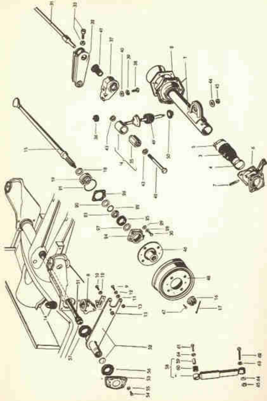
Fig. 23-V — Suspensão traseira da Variant. A do sedan é idêntica, apenas o tambor da roda (48) e o cubo (46) constituem uma só peça. (V. texto na pág. seguinte.)
