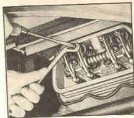
Fig. 3-F — Para firmar a regulagem, mantém-se o parafuso com a chave de fenda e aperta-se a contra-porca.
