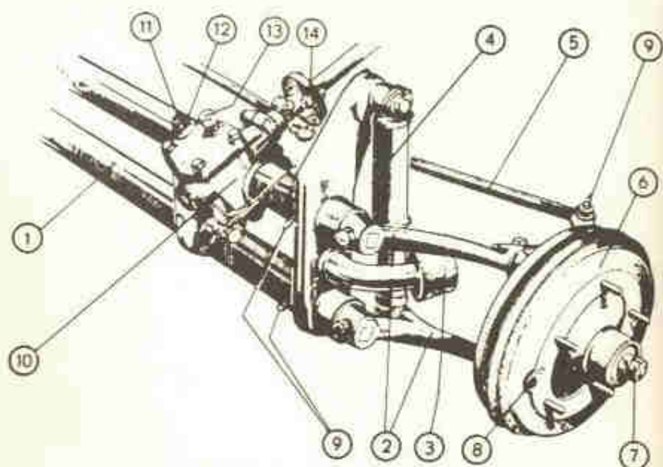
Fig. 1-L. — Parte esquerda da suspensão dianteira do sedan
