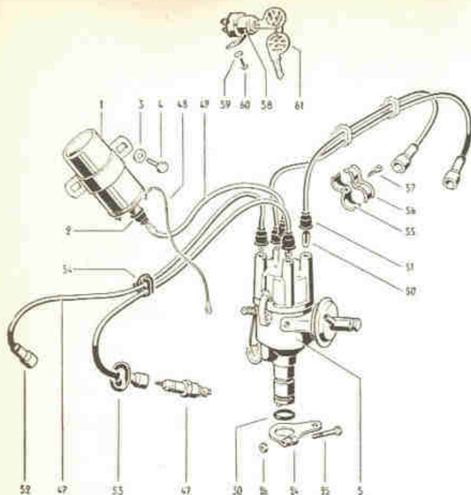
Fig. 1-D — Elementos do sistema de ignição
