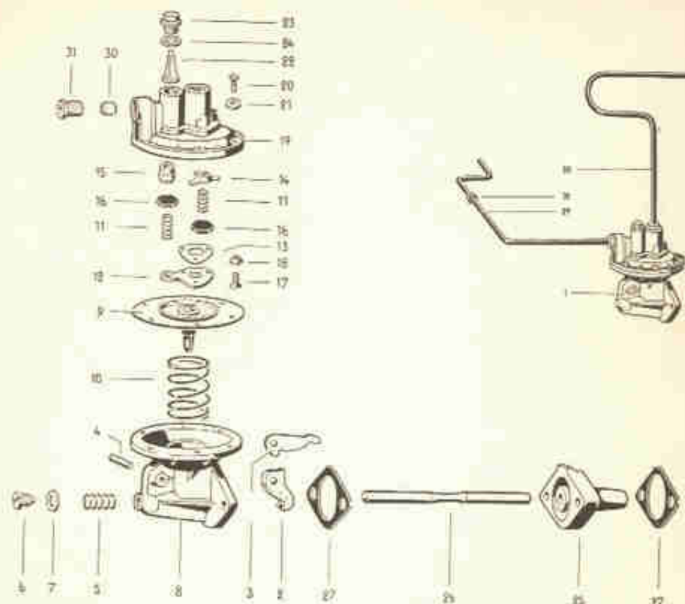
Fig. 3-E — A bomba de gasolina montada e desmontada (Motor "1200" — 36 HP)
