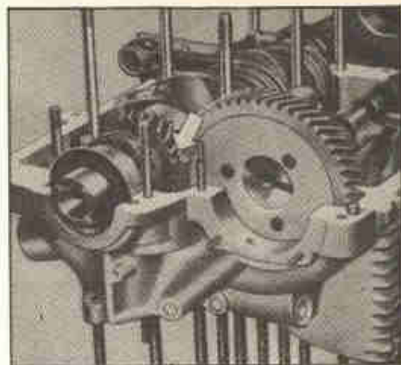
Fig. 8-H — Perfeito engraxamento da engrenagem da árvore de manivelas com a da árvore de comando de válvulas.
