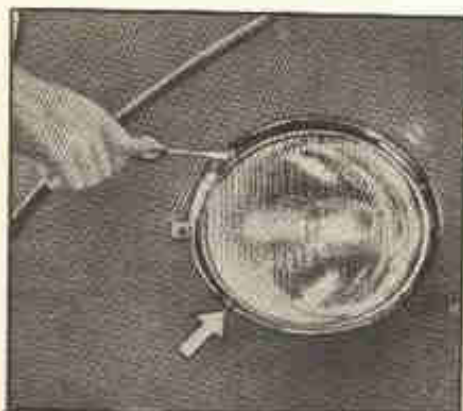
Fig. 13-S — Localização dos parafusos reguladores dos feixes dos faróis dos utilitários.
