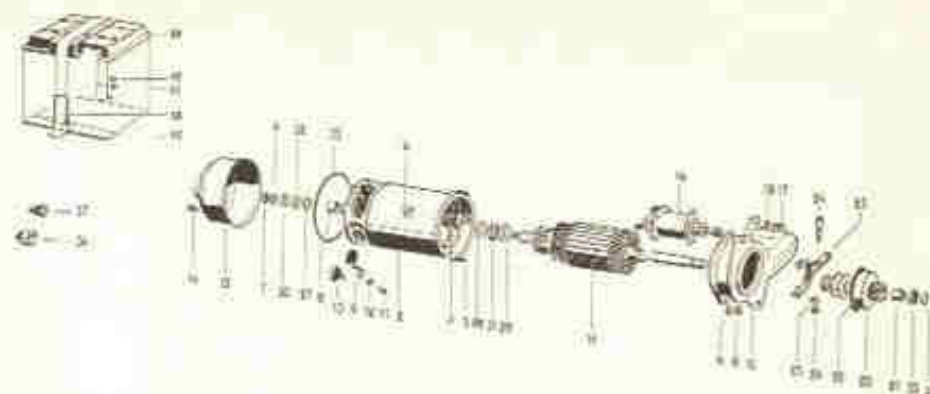
Fig. 10-S — O motor de partida Bosch desmontado e a caixa da bateria
