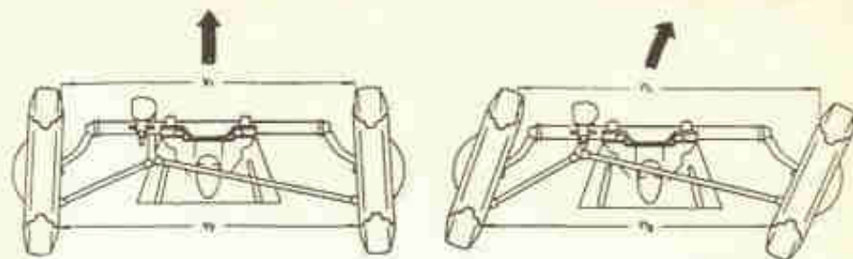
Fig. 3-Q — Ângulos de convergência e divergência nas curvas
