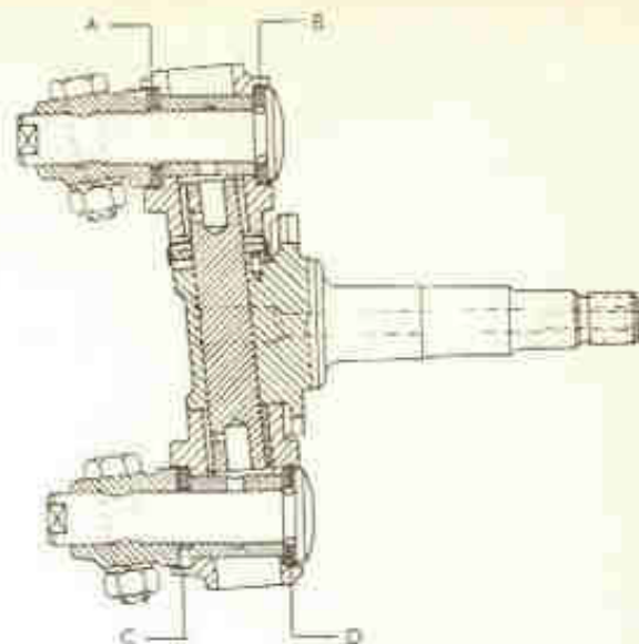
Fig. 9-N — Localização das arruelas de regulação dos pinos da suspensão (sedan e Karmann Ghia).
