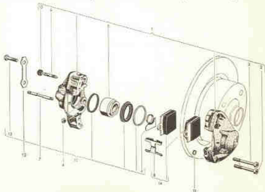
Fig. 24-V — Componentes do freio a disco do sedan "1600": 1 — Cavalete fixo do freio a disco; 2, 3 — Parafusos cilíndricos; 4 — Porca sextavada; 5 — Êmbolo de 40 mm; 6 — Chapa de retenção do êmbolo esquerdo; 7 — Pino de fixação das sapatas; 8 — Mola de retenção das sapatas; 9 — Parafuso de sangria; 10 — Coifa de proteção do parafuso de sangria; 11 — Junta; 12 — Chapa de segurança; 13 — Parafuso sextavado; 14 — Jogo de sapatas ("pastilhas") do freio a disco; 15 — Jogo de vedação do freio a disco.
