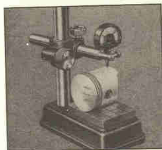
Fig. 17-H — A medida do diâmetro do êmbolo deve ser feita como mostra a ilustração ao lado: na parte inferior da sala.
