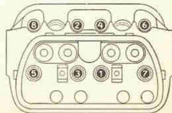
Fig. 5-H — Seqüência do apêto final das porcas do cabeçote.
