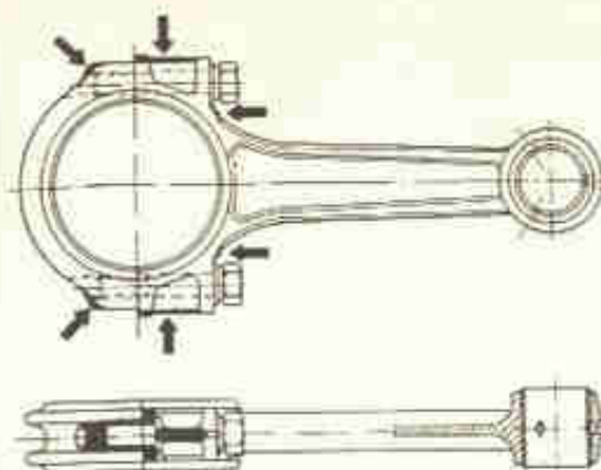
Fig. 21-H — As setas indicam os pontos da biela que podem ser retocados para igualar os pesos.
