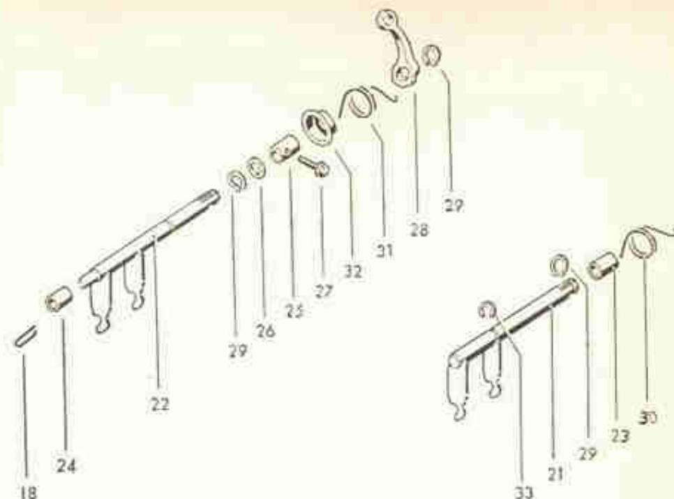
Fig. 3-1 — O garfo da embreagem e peças anexas.
