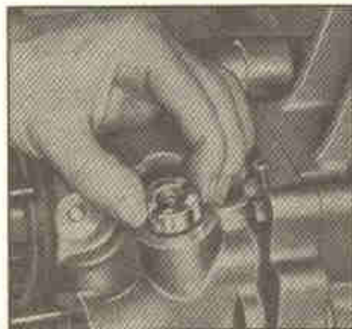
Fig. 31-H — Reposição da árvore de comando do distribuidor. Coloca-se o dedo no furo da vela n.º 1 e gira-se lentamente o motor até que se sinta a compressão ir aumentando; no final da compressão o cilindro está em ponto de combustão. Coloca-se provisoriamente a polia e então o entalhe deve coincidir com a junção das carcacas. (Fig. 30-D, pág. 33). Coloca-se a árvore com o entalhe superior paralelo ao plano da polia e com o lado mais estreito do excêntrico voltado para a mesma.
