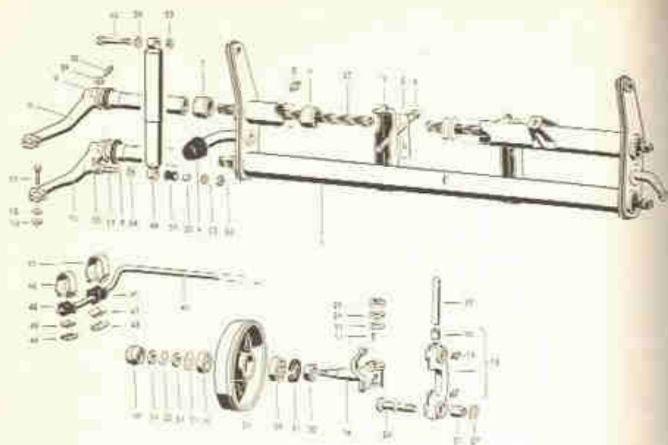
Fig. 2-L — Suspensão dianteira do sedan e do Karmann Ghia
