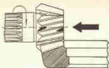
Fig. 24-J — Fresagem Klingelnberg. Marcas deixadas nos dentes do pinhão:
