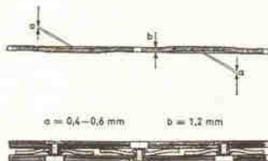
Fig. 5-I — Concavidade das molas do disco da embreagem (a) e sua espessura (b). — Na ilustração de baixo, vemos como rebitar as guarnições.
