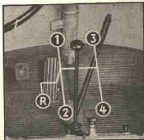
Fig. 5-T — As 5 posições da alavanca de mudanças.
