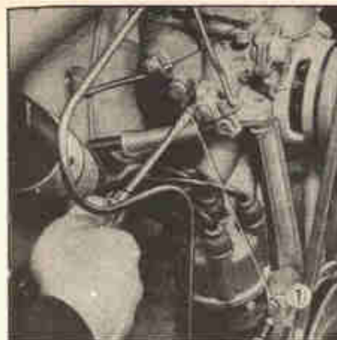
Fig. 17-E — Regulagem da mistura de marcha-lenta.
