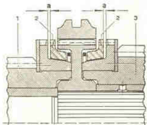
Fig. 9-J — Corte do sincronizador de 3. a e 4. a velocidades.
