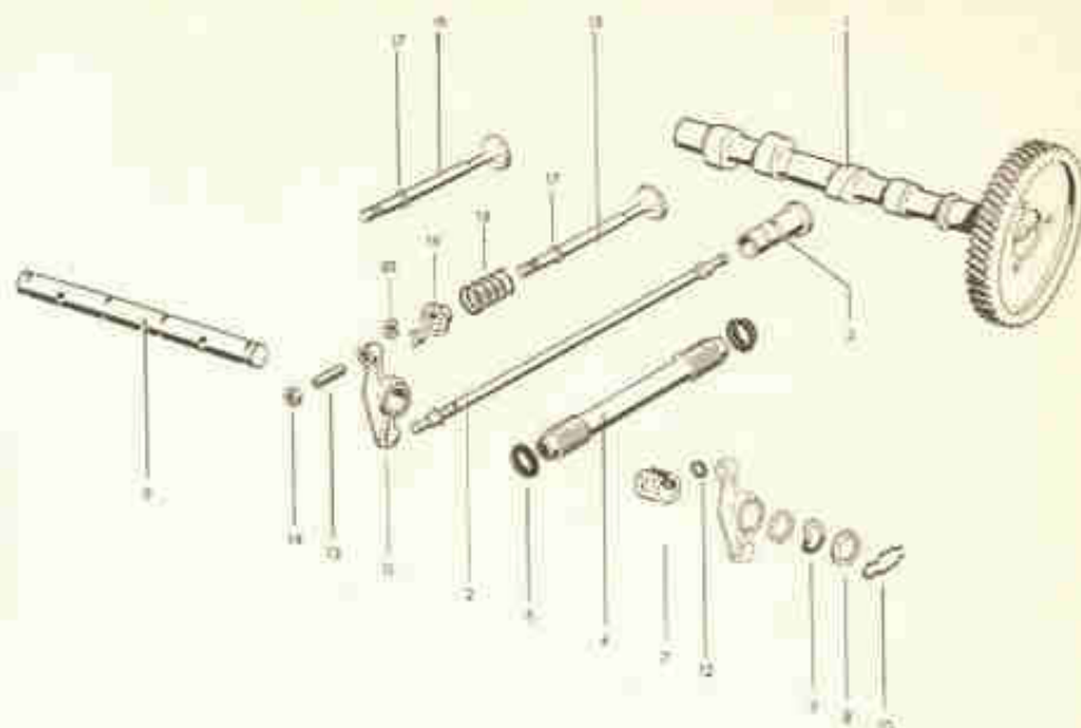
Fig. 27-H — Peças do mecanismo de válvulas ("1300", "1500", "1600" e "1600" plano).
