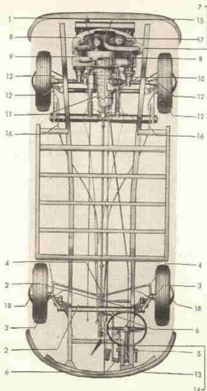
Plano de lubrificação dos utilitários
