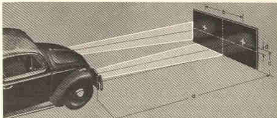
Fig. 12-S — Regulagem dos faróis
