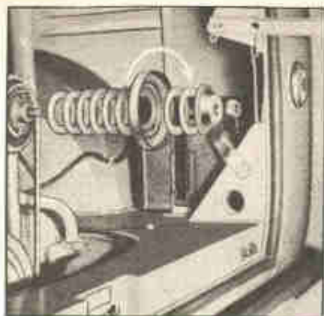
Fig. 3-B — Localização das arruelas de ajuste da correia.
