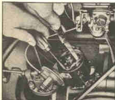
Abertura dos platinados: 0,4 mm (Todos os modelos)
