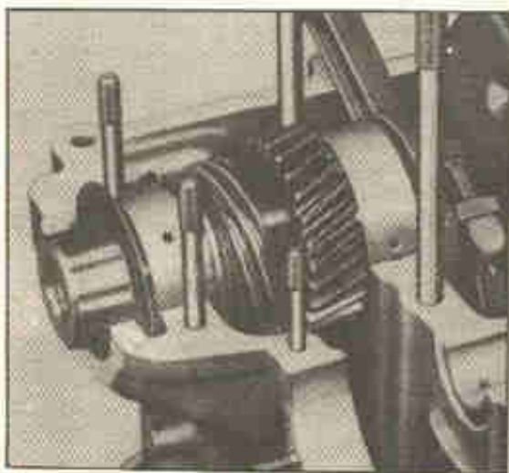
Fig. 10-H — Detalhe de montagem da árvore de manivelas, mostrando o anel defletor de óleo no lugar.
