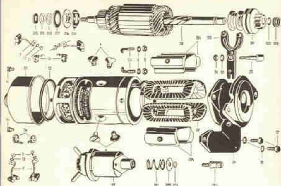
Fig. 11-S — O motor de partida Walita, desmontado
