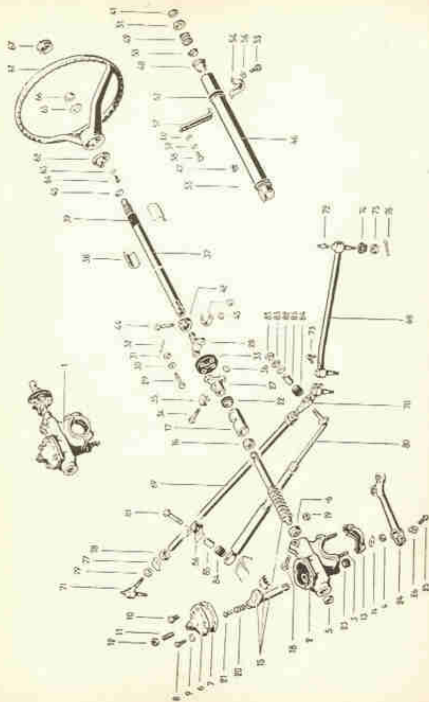
Fig. 1-N — Sistema de direção do sedan e do Karman Ghia 1962-63. Os modelos anteriores não possuem o amortecedor de direção e apresentam pequenas diferenças, conservando, no entanto, a estrutura básica.
