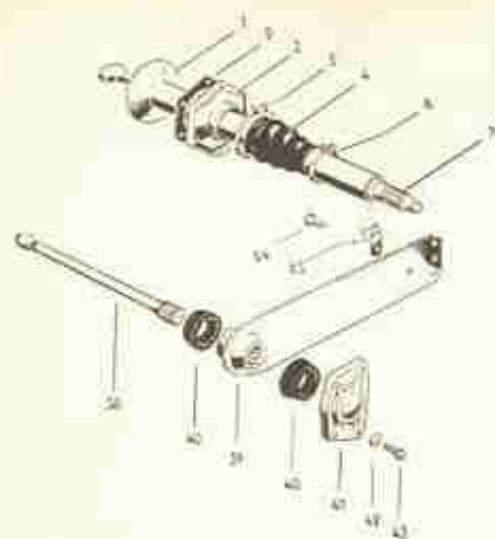
Fig. 2-M — Parte da suspensão traseira dos utilitários. (V. restante à pág. 114).
