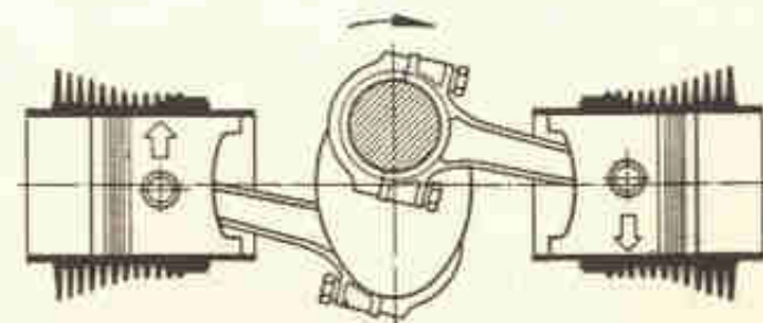
Fig. 2 — Disposição dos cilindros do motor Volkswagen
