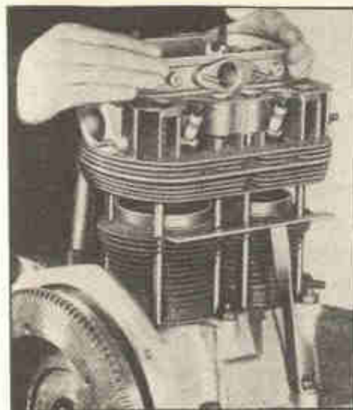
Fig. 30-H — Reposição do cabeçote. As duas juntas entre os cilindros e o cabeçote já se encontram no lugar. Vê-se que essas juntas não se encontram entre as superfícies de contato dessas peças, mas um pouco mais abaixo.
