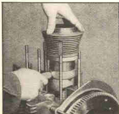
Fig. 23-H — A reposição dos cilindros se faz facilmente com auxílio da cinta de compressão de anéis VW 123 a, como mostra a figura ao lado.
