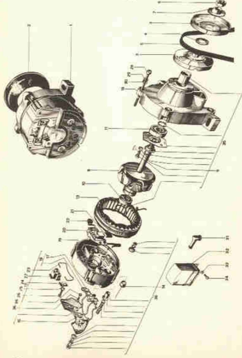
Fig. 31-V — O alternador inteiramente desmontado.
