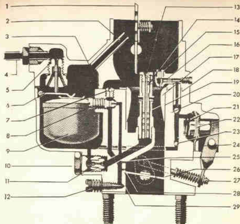
Fig. 7-E — Corte do carburador 28 PCI
