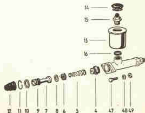
Fig. 5-R — Cilindro mestre dos utilitários desmontado.
