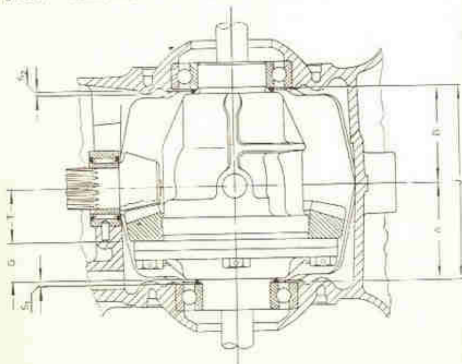
Fig. 15-J — Medidas necessárias para ajuste do diferencial. As ilustrações desta página mostram o diferencial do sedan. No da Kombi as marcações e medidas são as mesmas, mas a coroa se situa do lado direito.
