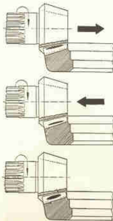
Fig. 23-J — Impressões deixadas nos dentes da coroa pela tinta aplicada no pinhão. (Fresagem Gleason).
