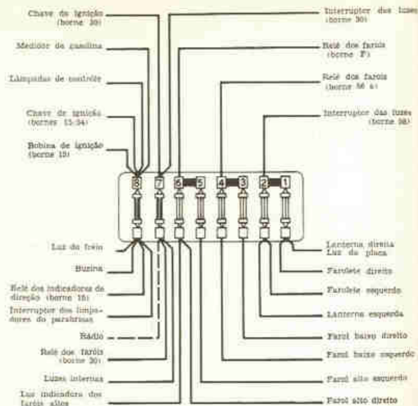
Fig. 5-S — Caixa de fusíveis do sedan "1300"
