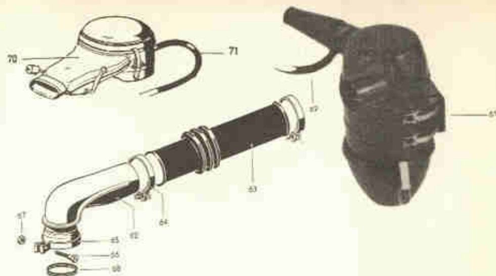
Fig. 19-E — Filtros de ar dos modelos "1300", "1500" e sedan "1600".
