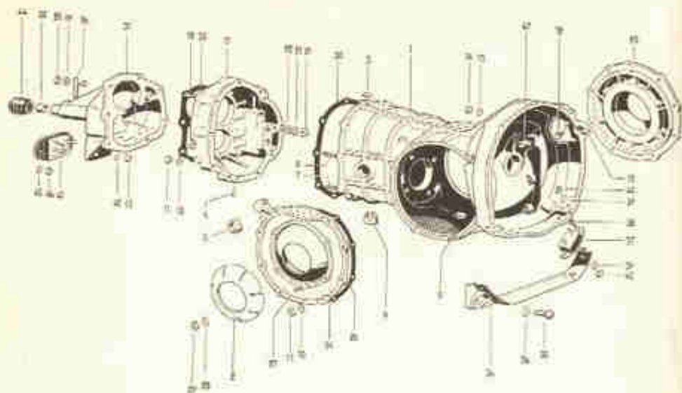
Fig. 2-K — Carcaça da transmissão e peças anexas
