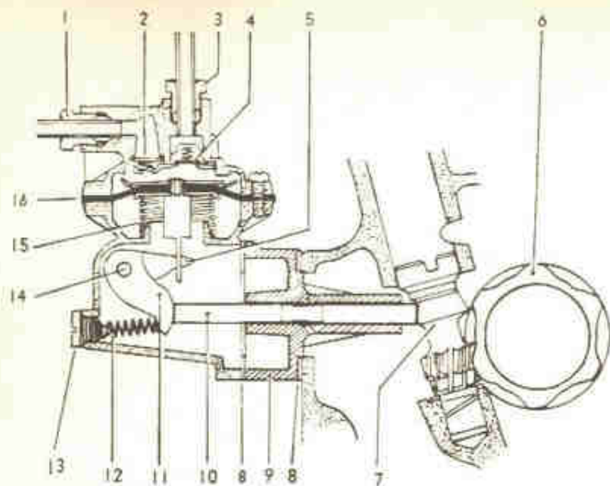
Fig. 2-E — Corte da bomba de gasolina. (Motor "1200" — 36 HP)
