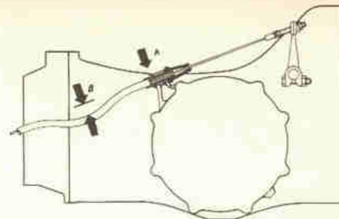
Fig. 11-1 — Detalhes do cabo de comando da embreagem, modelos com caixa de mudanças totalmente sincronizada. Nos modelos com caixa de mudanças parcialmente sincronizada a diferença reside no suporte do conduíte, que tem outra forma.
