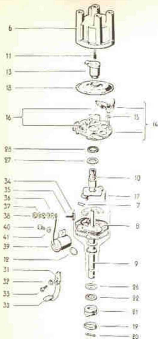
Fig. 3-D — Distribuidor da Kombi "1200" — 36 HP, inteiramente desmontado. Os demais elementos do sistema de ignição da Kombi são os mesmos mostrados na fig. 1-D, excepto no que se refere ao avanço a vácuo que a Kombi "1200" não possui.
