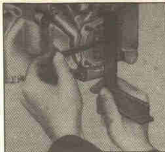
Fig. 32-H — Medida da folga axial das engrenagens da bomba. Com as juntas, essa folga deve estar compreendida entre 0,066 e 0,183 (sem aperto inicial). Veja a pág. 22.
