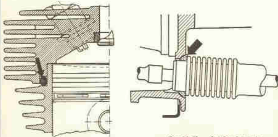
Fig. 29-H — O tubo de proteção da vareta do tucho possui duas juntas uma entre o tubo e a carcaça do motor e outra entre o tubo e o cabeçote.
