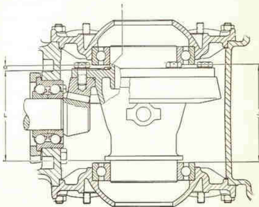
Fig. 12 — Medidas necessárias para o ajuste da coroa.
