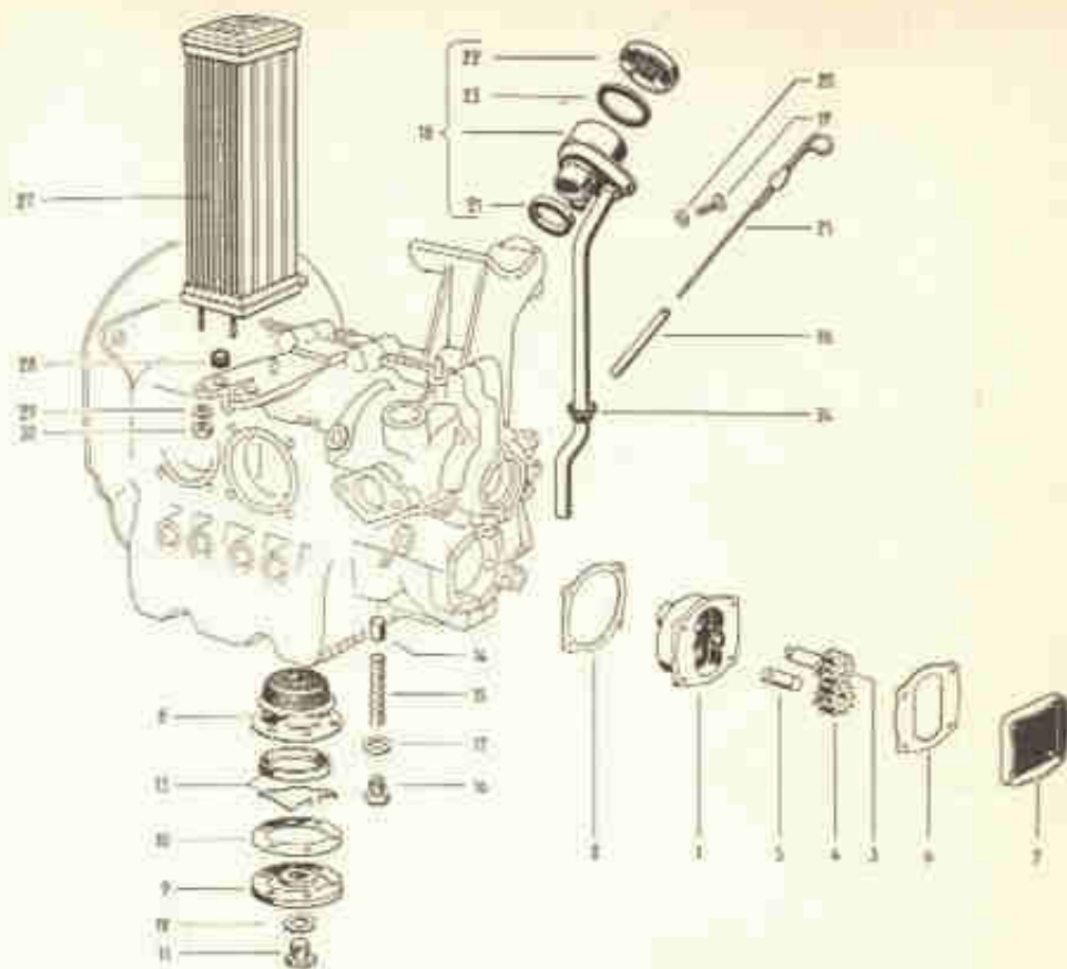
Fig. 1-C — O sistema de lubrificação desmontado.
