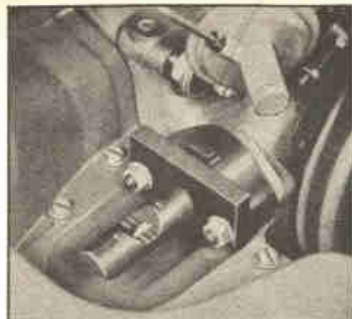
Fig. 6-E — Na ilustração ao lado vê-se como colocar o dispositivo próprio para medir o curso do pino de comando. (Motor "1200" — 16 HP). (Calibre VW 328 a)
