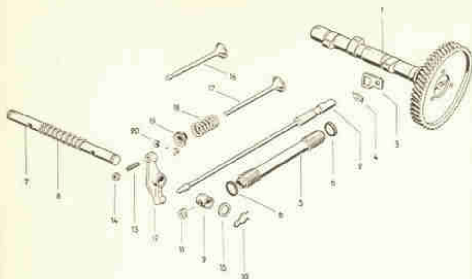
Fig. 26-H — Peças do mecanismo de válvulas. ("1300" — 36 HP)
