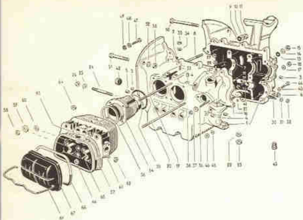
Fig. 2-H — O motor "1200" desmontado mas sem os principais órgãos móveis
