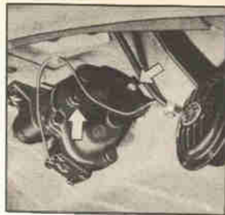
Fig. 4-P — A seta superior indica o bujão de abastecimento da caixa de direção e a inferior, o parafuso de regulagem da folga axial. Nos modelos recentes o bujão de abastecimento se encontra na parte frontal da caixa.
