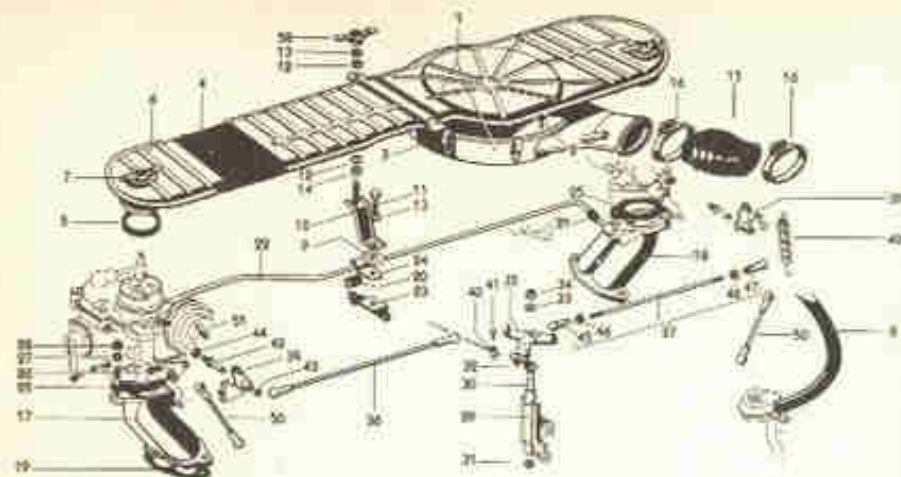
Fig. — 10-V — Sistema de admissão do motor da Variant.
