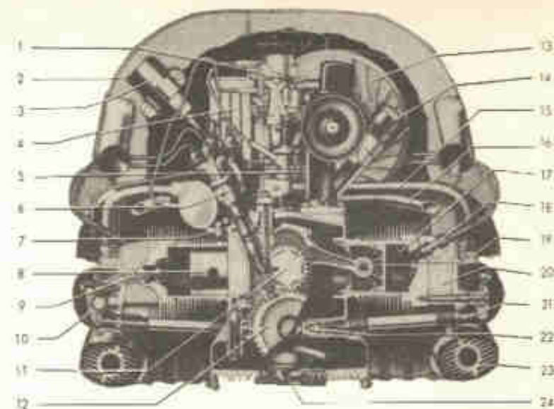
Fig. 3-A — Corte do motor "1 300" por um plano vertical paralelo aos cilindros. Os motores "1 500" e "1 400" são semelhantes; diferem apenas nos diâmetros dos cilindros e em pequenos outros detalhes.
