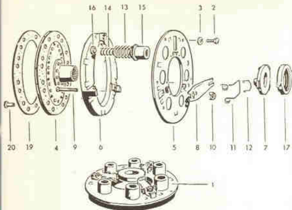
Fig. 2-1 — A embreagem montada (1) e suas partes constituintes destacadas. A ilustração acima foi retirada do catálogo de peças da Kombi, mas as diferenças entre todos os modelos residem em medidas e detalhes de construção, como se segue. Nos modelos de 36 HP (até 1966) o sedan e o Karman Ghia possuem colar de carvão, que pode ser substituído pelo tipo de rolamento, usado nos utilitários, desde que se troquem também as molas de retenção. Os modelos "1300" e "1500" são todos equipados com colar de rolamento. Em todos os modelos, os utilitários possuem duas molas de pressão, uma interna (14) e outra externa (13) em cada conjunto. O sedan e o Karman Ghia possuem somente uma mola de pressão, em todos os modelos. Nos modelos "1300" e "1500" a regulagem do platô se faz por meio das porcas, pois os parafusos são oscilantes e todo o conjunto é mais reforçado que o anterior.
