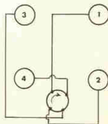
Fig. 8-V — Numeração dos cilindros e ordem de explosão (1-4-3-2)
