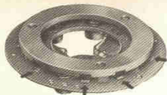
Fig. 6-I — Ao se colocar a embreagem no volante, as saliências que centram a tampa, indicadas pelas setas, devem se alojar devidamente no volante. Os parafusos que fixam o suporte do plato ao volante devem ser apertados gradativamente e alternando os diametralmente opostos. O aperto final deve ser de 4 kgm.
