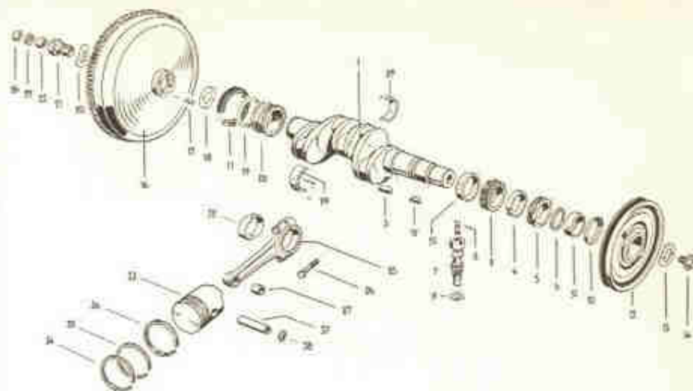
Fig. 6-H — Principais órgãos móveis do motor "1200" — 36 HP
