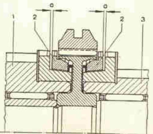
Fig. 9-K — Corte do sincronizador de 3. a e 4. a velocidades.
