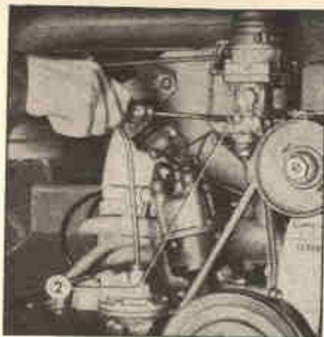
Fig. 16-E — Regulagem da velocidade de marcha-lenta.
