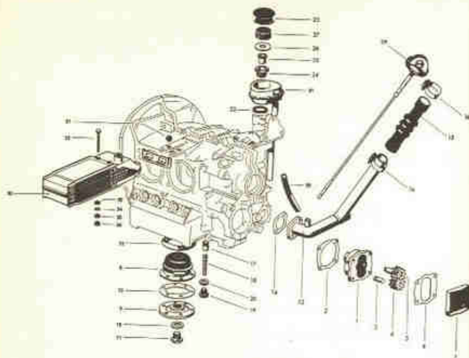
Fig. 6-V — Sistema de lubrificação do motor plano "1600".
