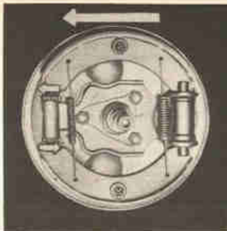
Fig. 8-R — Prato de freio das rodas dianteiras do sedan e do Karmann Ghia, mostrando a localização dos reguladores. As setas menores indicam o sentido em que os reguladores devem ser girados para aproximar as sapatas do tambor. A seta maior indica a frente do carro. Nos modelos alemães antigos, os reguladores se situam na parte superior, ligeiramente inclinados para a frente.
