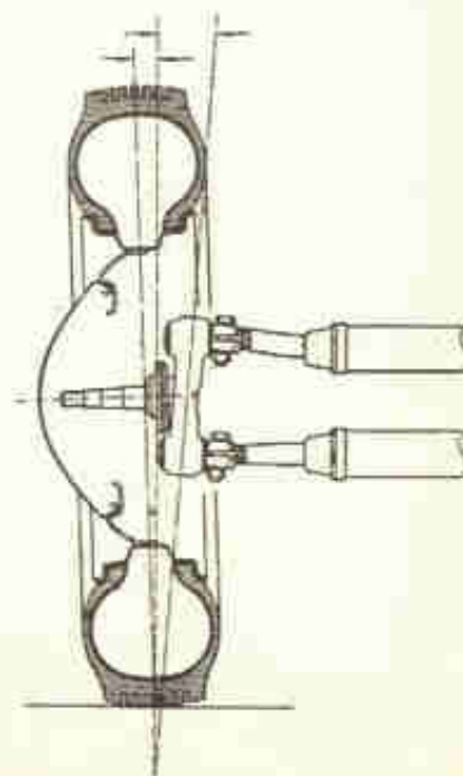
Fig. 1-Q — \alpha — Queda da roda \mu — Inclinação do pino mestre
