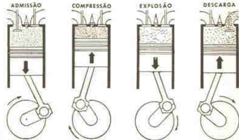
Fig. 1 — As 4 fases do ciclo a 4 tempos
