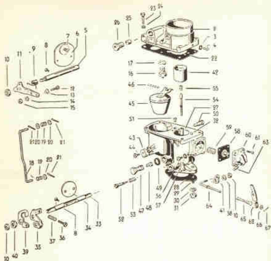
Fig. 13-E — O carburador inteiramente desmontado. (Motor "1200" — 36 HP)
