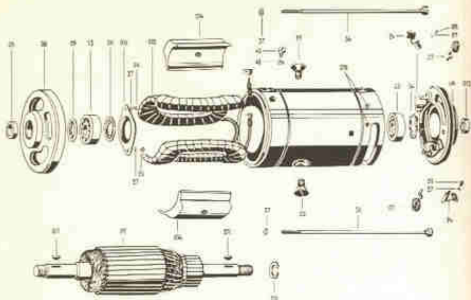
Fig. 8-S — O dinamo "Walita" inteiramente desmontado
