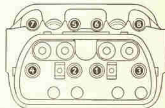
Fig. 4-H — Seqüência de apêto inicial das porcas do cabeçote.
