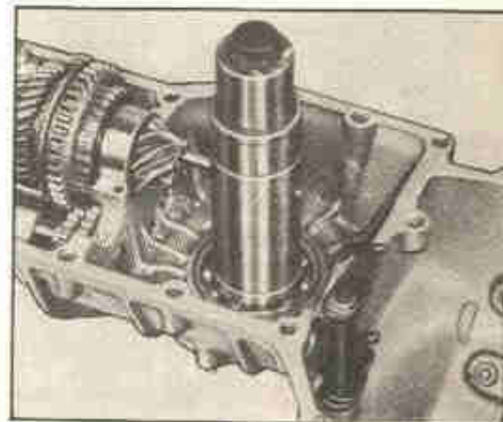
Fig. 16-J — O calibre VW 289 b colocado no anel interno do rolamento esquerdo do diferencial.
