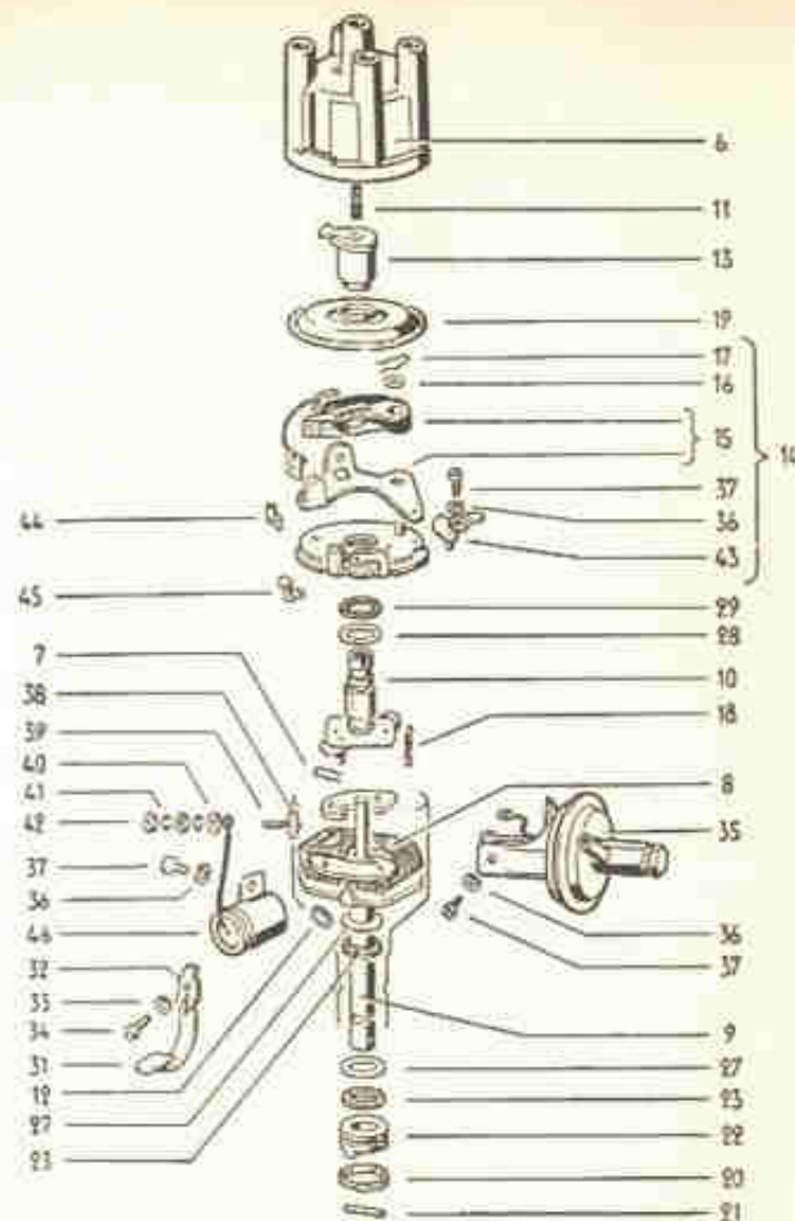
Fig. 2-D — O distribuidor inteiramente desmontado (sedan 36 HP)
